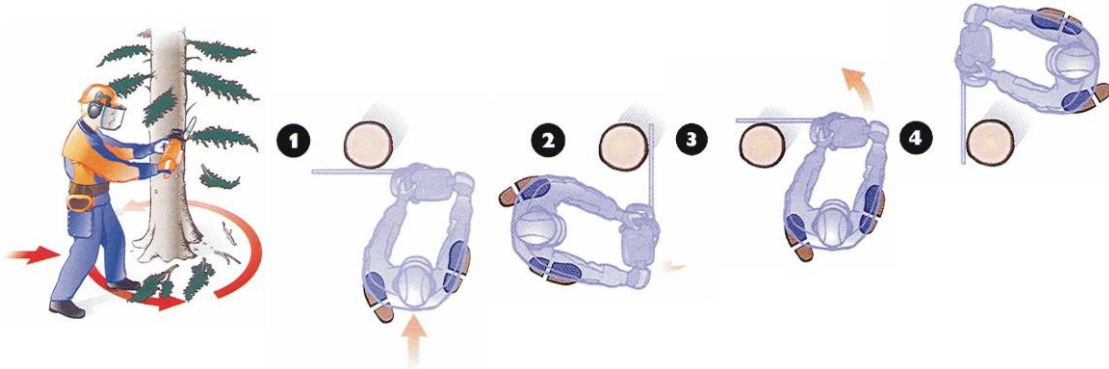
Rys.6 Technika podkrzesywania drzewa z zastosowaniem pilarki
