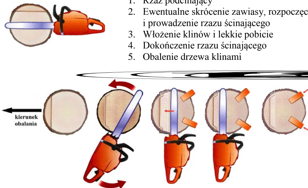
Rys.17 Technika ścinki i obalania drzewa o średnicy mniejszej od użytecznej długości prowadnicy
