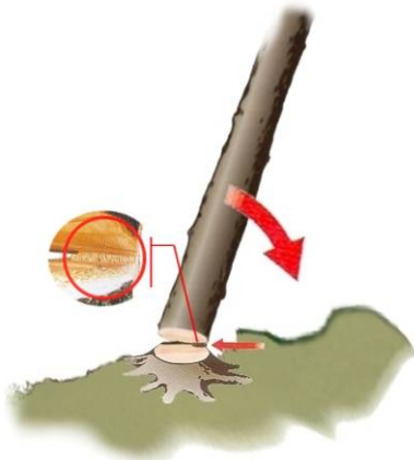
Rys.35 Obrót drzewa z wykorzystaniem fragmentu zawiasy Rys.36 Ściąganie drzewa z wykorzystaniem ślizgu.
