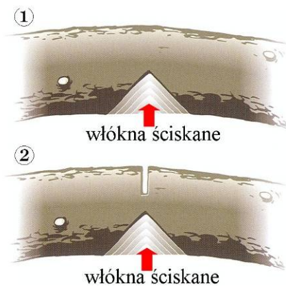
Rys.69 Cięcie drewna o dużych naprężeniach – rzaż w kształcie litery „V”.
