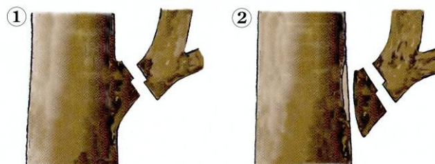
Rys.38 Technika odcinania grubych gałęzi.
