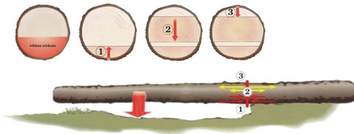
Rys.46 Technika przerzynki drewna mocno naprężonego.
